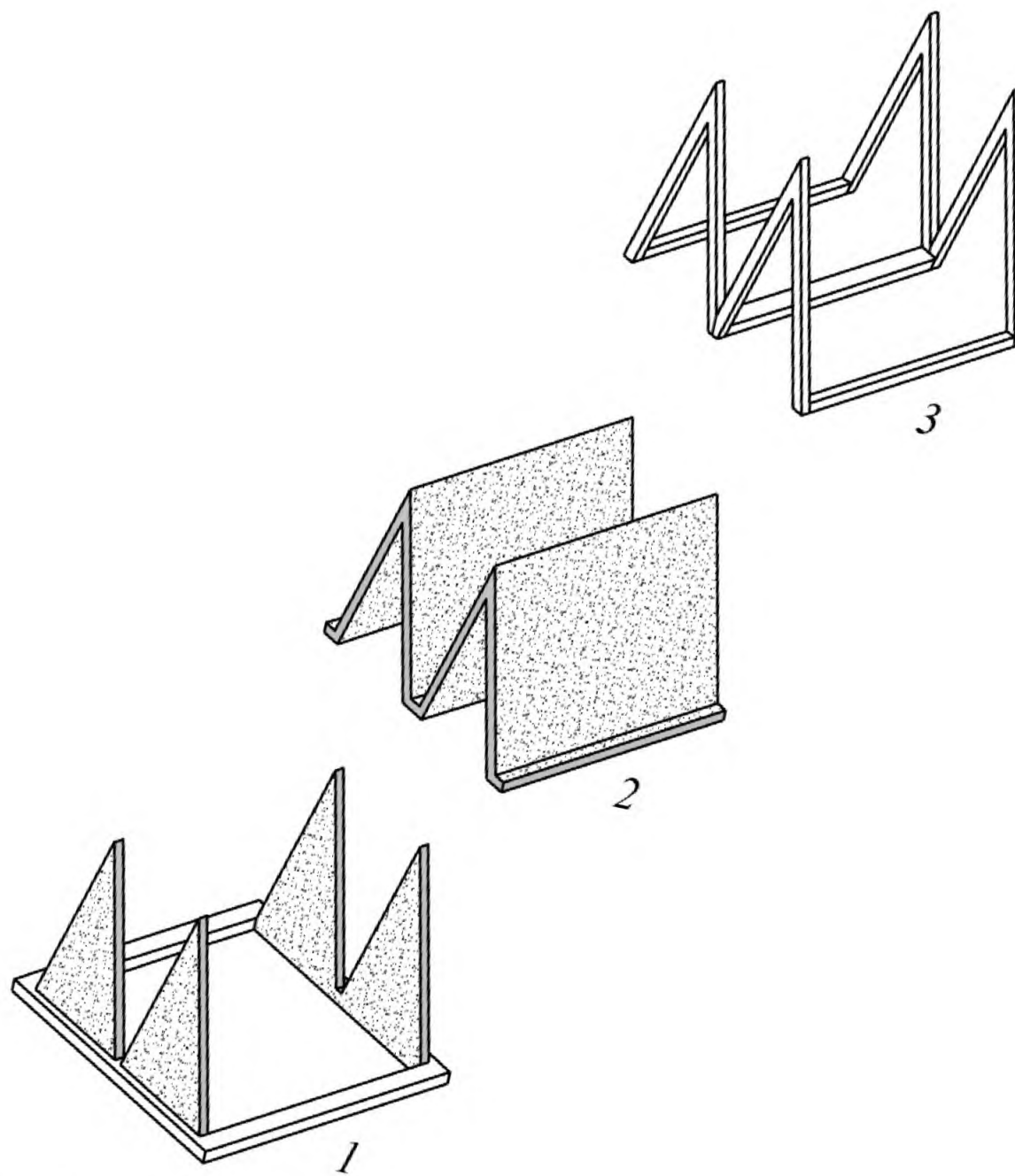
1 — рамка W-формы; 2 — фильтрующий материал ( 1 \text{ м}^2 ); 3 — прижимная рамка W-формы Рисунок В.1 — Пример рамки W-формы и деталей для испытаний фильтрующего материала
